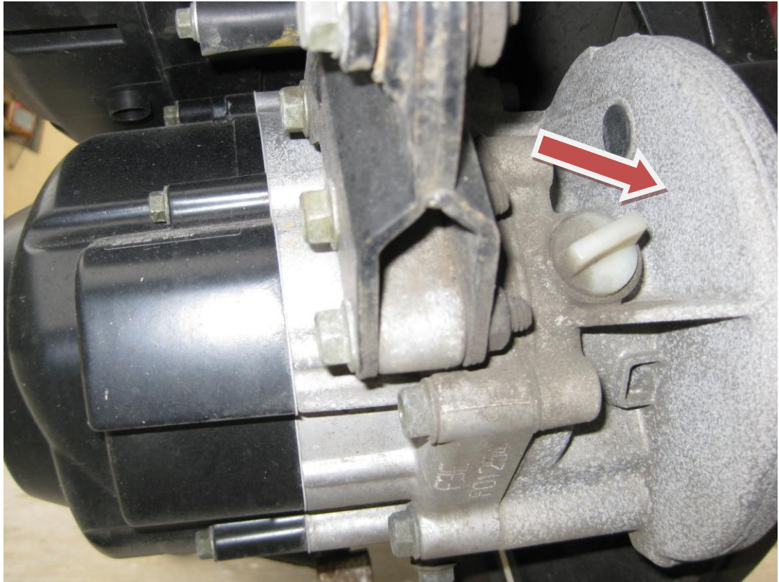
圖十、引擎 Case 鋁合金部份起白色氧化物，嚴重銹蝕（僅以清水洗車）
