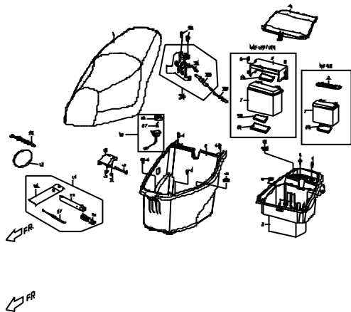
F10 座墊, 前置物箱, 後置物箱 SEAT.FR LUGGAGE. BACK LUGGAGE .
