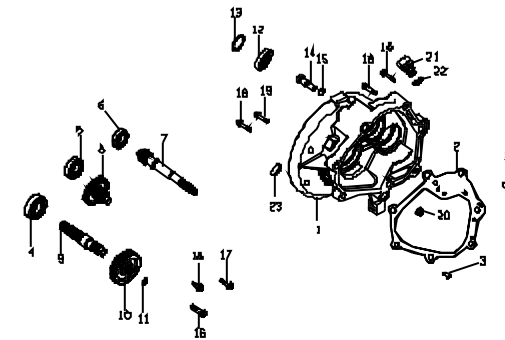
E10 傳動齒輪箱 GEAR TRANSMISSION
