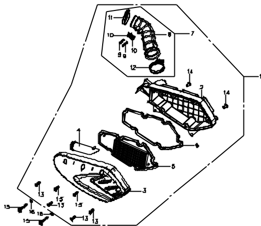
E11. 空氣濾清器組合(有EEC) AIR CLEANER COMP. W/H EEC SYSTEM
