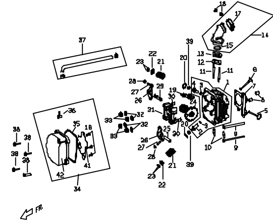
E3.1 汽缸頭 (125 CC) CYLINDER HEAD
