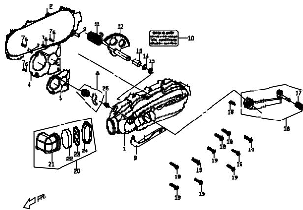
E2 左邊蓋 LH SIDE COVER
