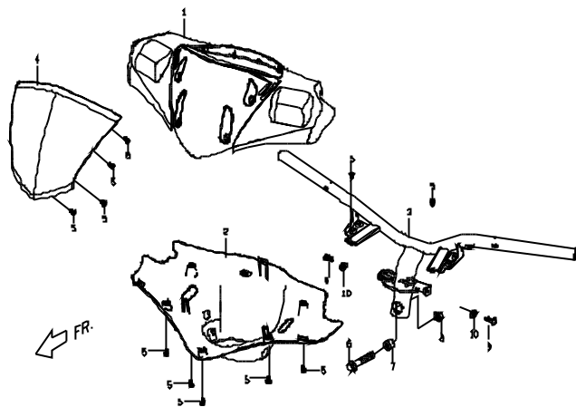
F1 方向把手前後蓋。方向把手管。遮陽板 COVER UPPER & LOWER HANDLE BAR. SUN PLATE.
