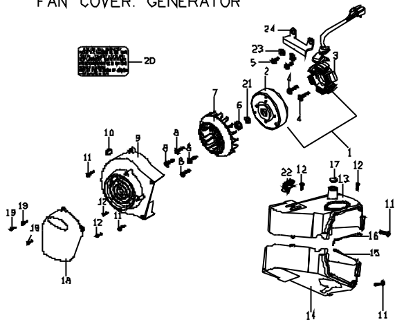
E8 發電機 / 風扇罩 FAN COVER, GENERATOR
