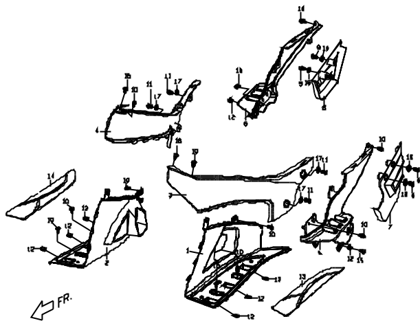
F7 腳踏版。 STEP FLOOR.STEP PLATE.
