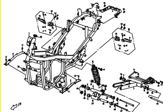
F12.2 車架 (125/150c.c) FRAME
