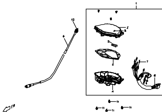
F2 碼錶 SPEEDOMETER
