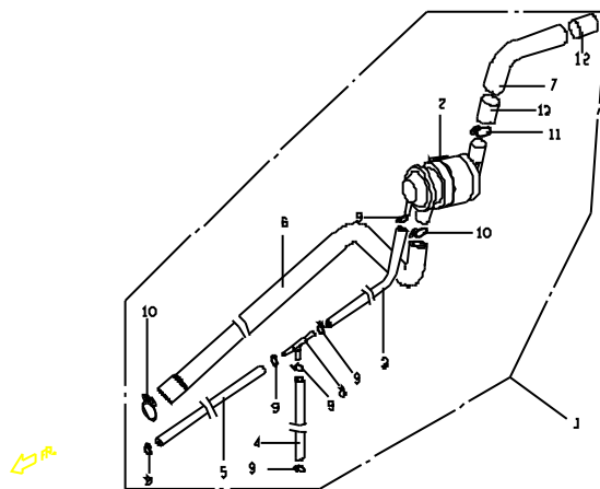
E15 空氣導入控制閥總成 AIAC ASSY. (OPTIONAL DEVICE)
