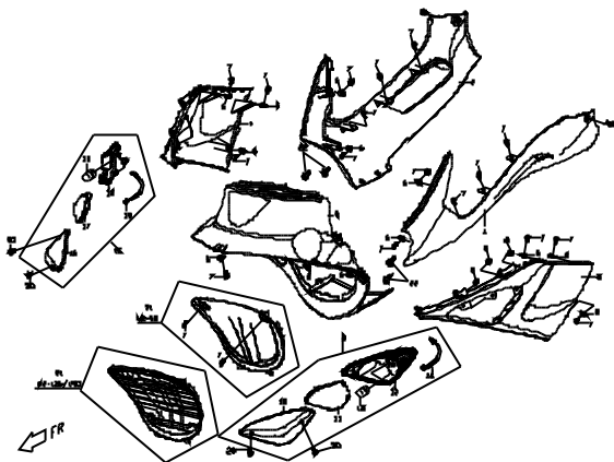
F8 前下蓋, 腳踏板下腹蓋, 前土除 FRT LOWER COVER.STEPFLOOR LOWER COVER.FRONT FENDER
