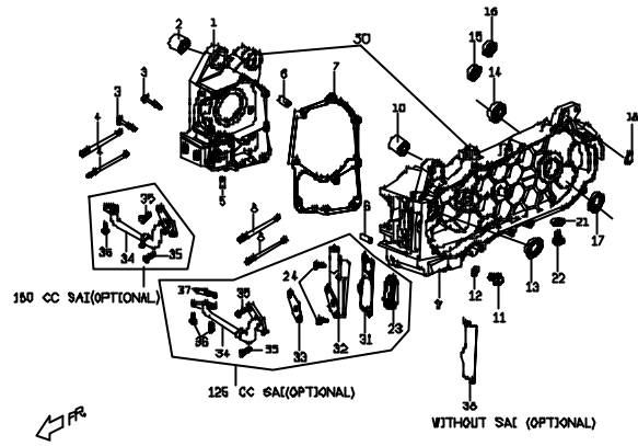
E1 曲軸箱 CRANK CASE
