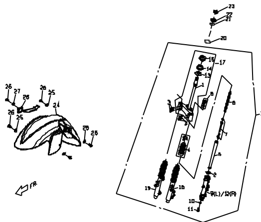
F 4.2 前叉 (125/150CC) FRONT FORK
