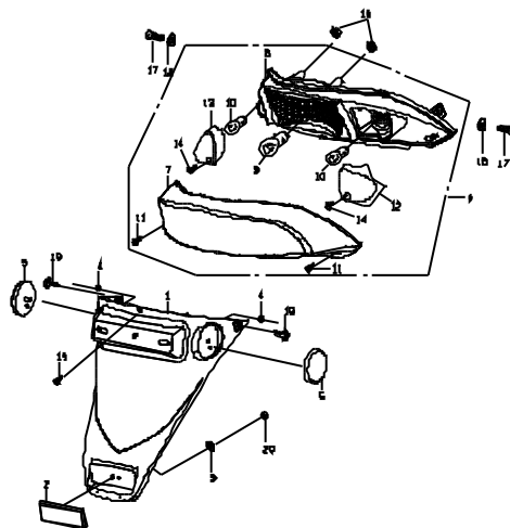
F11 牌照板, 反光片, 後燈。 LICENSE PLATE.REFLECTOR. BACK LAMP.
