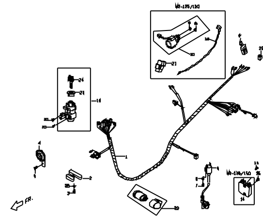
F15.2 主配線 M2-125/150 WIRE HARNESS
