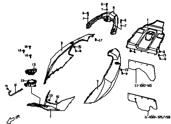
F9 車身蓋, 中間蓋, 後行李架, 車身下腹蓋。 BODY COVER.MIDDLE COVER. RR LUGGAGE.BODY LOWER COVER.
