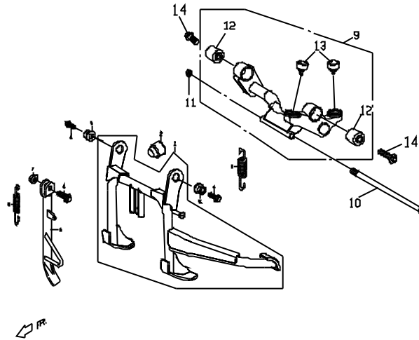
F14.2 中腳柱, 側腳柱 CENTER STAND, SIDE STAND
