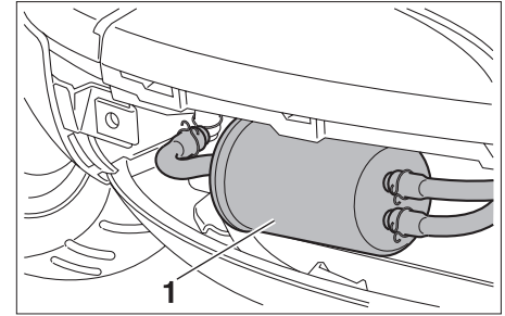
1. 活性碳罐
