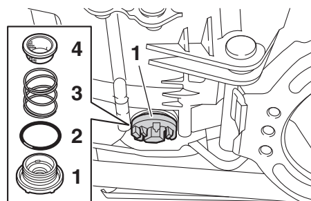
1. 排油螺栓B 2. 護油圈
