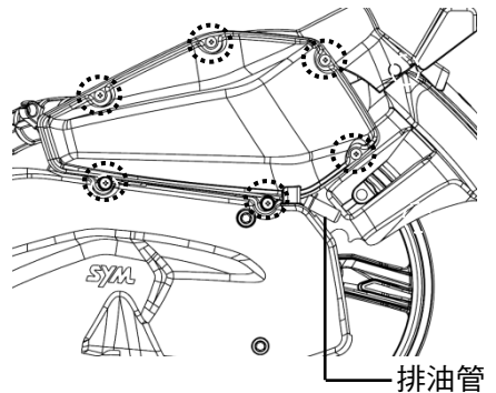
濾清器外蓋固定螺絲
