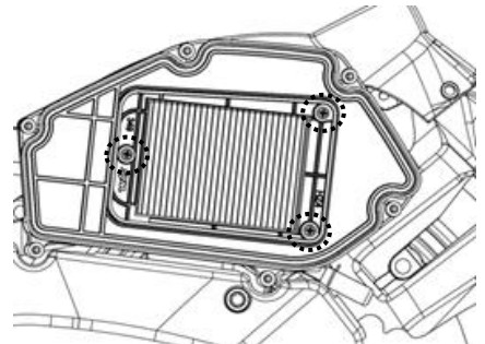
濾清器濾芯固定螺絲
