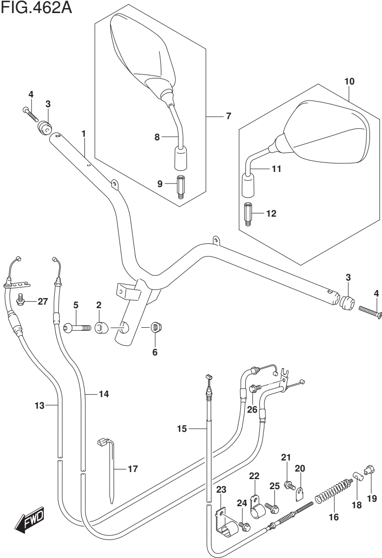
FIG. 462A (1-D-14) ハンドルバー (UG125SEBL9)
