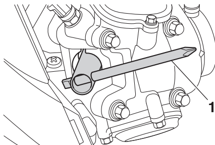
1. 火星塞扳手
