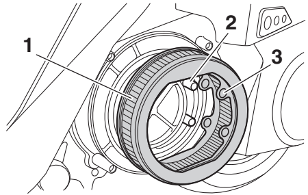
1. 濾清器濾蕊
