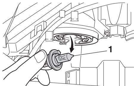
1. 前燈燈泡
