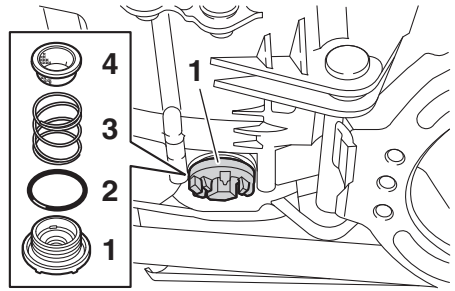
1. 排油螺栓B 2. 護油圈
