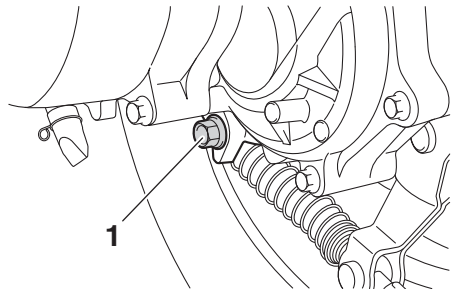
1. 排油螺栓
