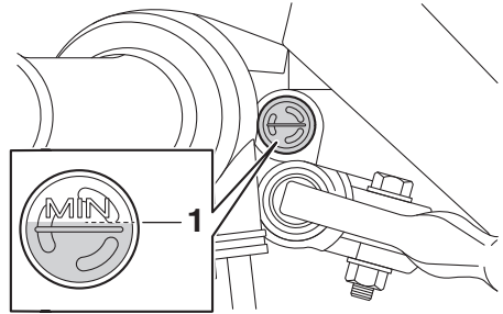
1. 下限記號
