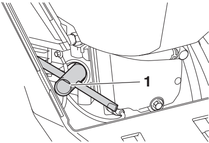
1. 火星塞扳手
