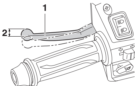
1. 後煞車把手 2. 自由間隙
