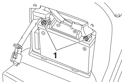
1. 固定螺栓(X2)
