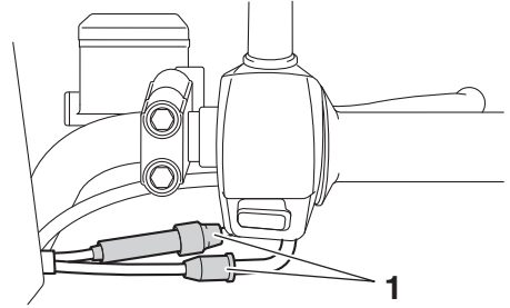
1. 防塵橡皮套
