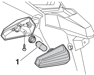
1. 後方向燈
