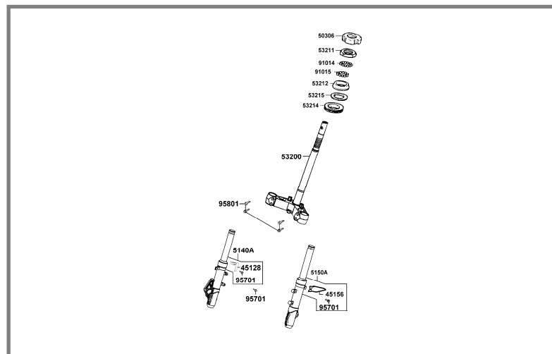
F06 TIJA DIRECCION (Pág. 77)
