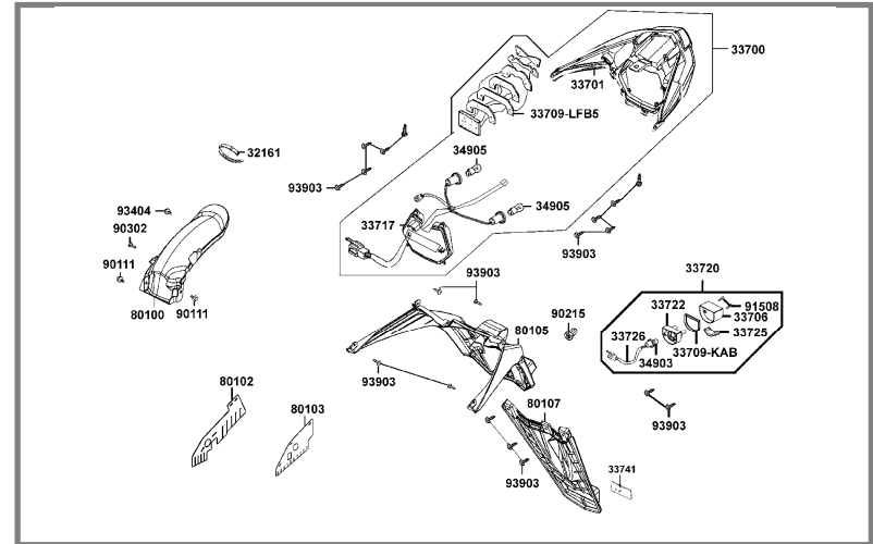
F18 GBARROS/PILOTO TRASERO (Pág. 115)
