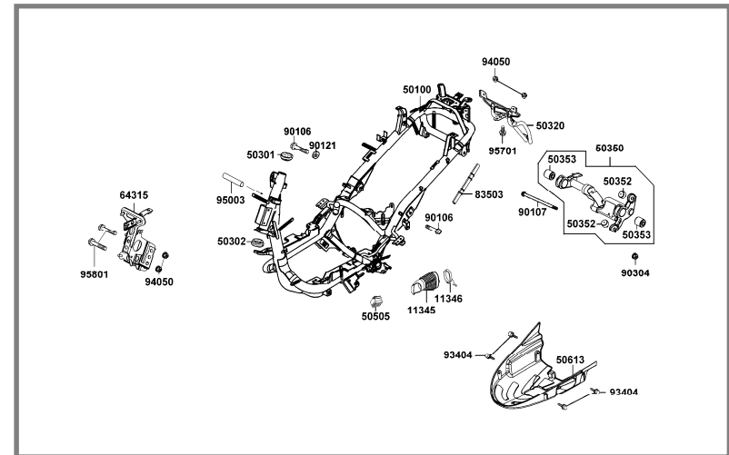
F20 CHASIS (Pág. 124)
