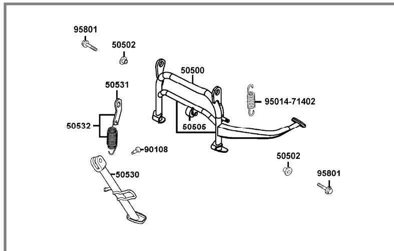
F15 CABALLETES (Pág. 109)
