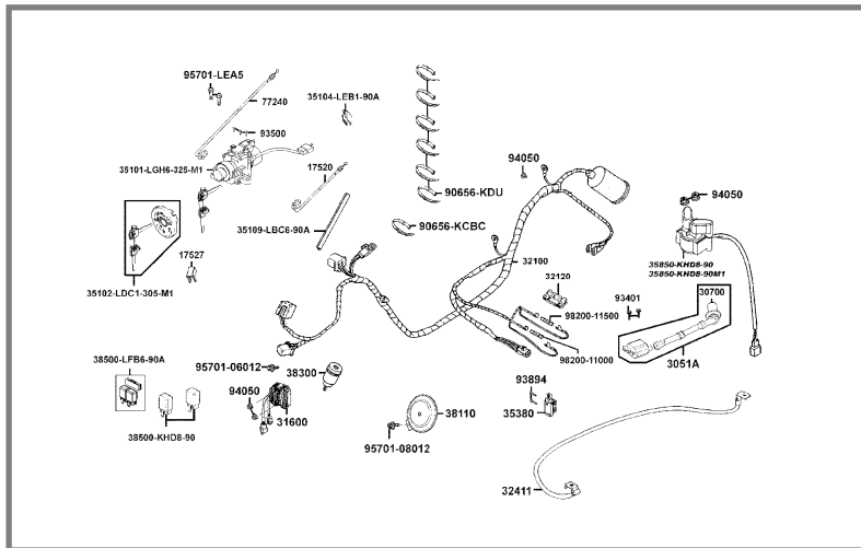
F19 INSTALACION ELECTRICA (Pág. 119)
