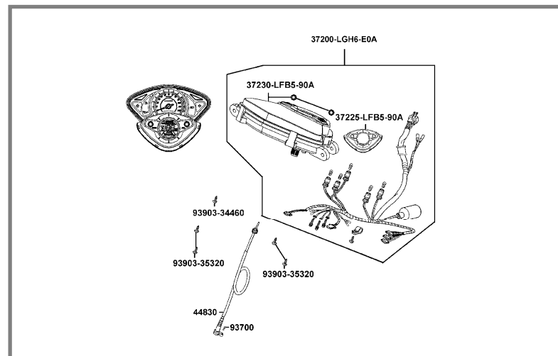
F02 VELOCIMETRO (Pág. 59)
