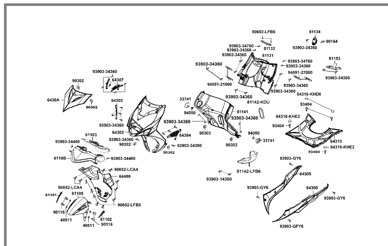
F05 CARROCERIA DELANTERA (Pág. 71)
