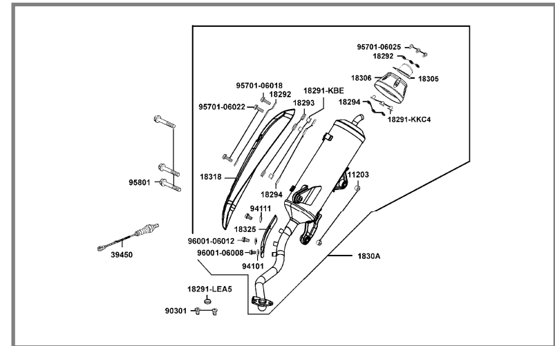
F14 ESCAPE (Pág. 105)
