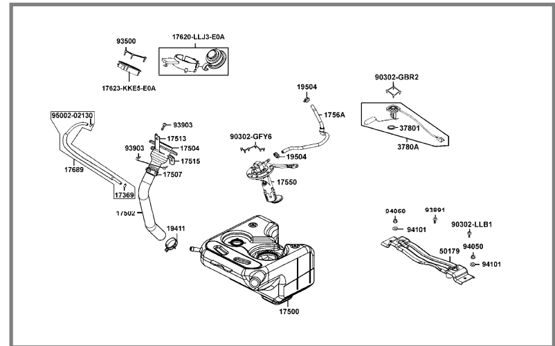
F10 DEPOSITO DE GASOLINA (Pág. 91)
