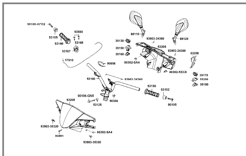
F03 MANILLAR - ESPEJOS (Pág. 61)
