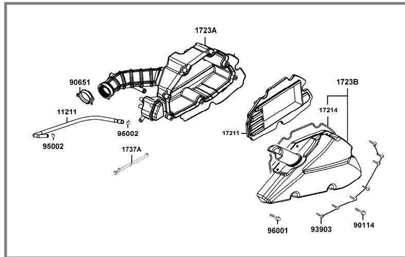
F13 FILTRO DE AIRE (Pág. 101)
