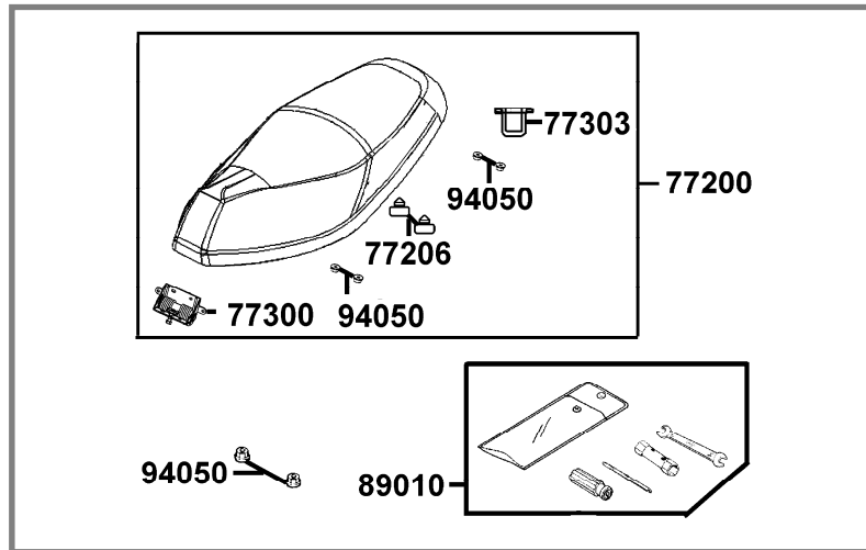
F09 ASIENTO (Pág. 89)
