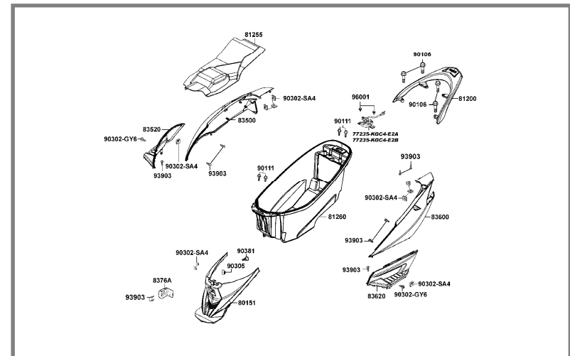
F12 CARROCERIA TRASERA (Pág. 97)
