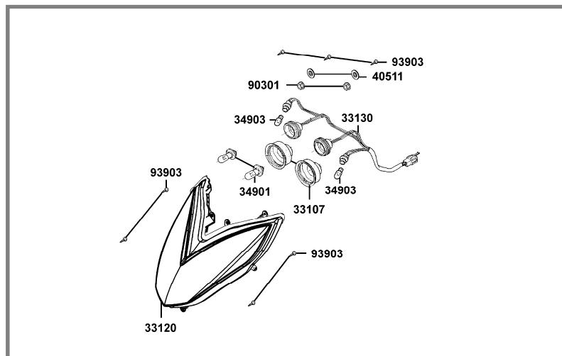
F01 FARO DELANTERO (Pág. 57)
