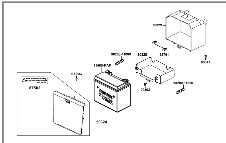
F11 BATERIA (Pág. 95)
