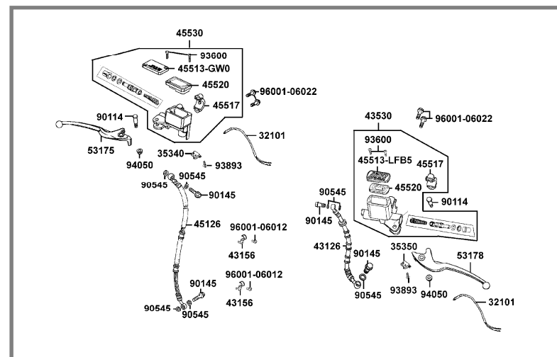
F04 BOMBAS DE FRENO (Pág. 67)
