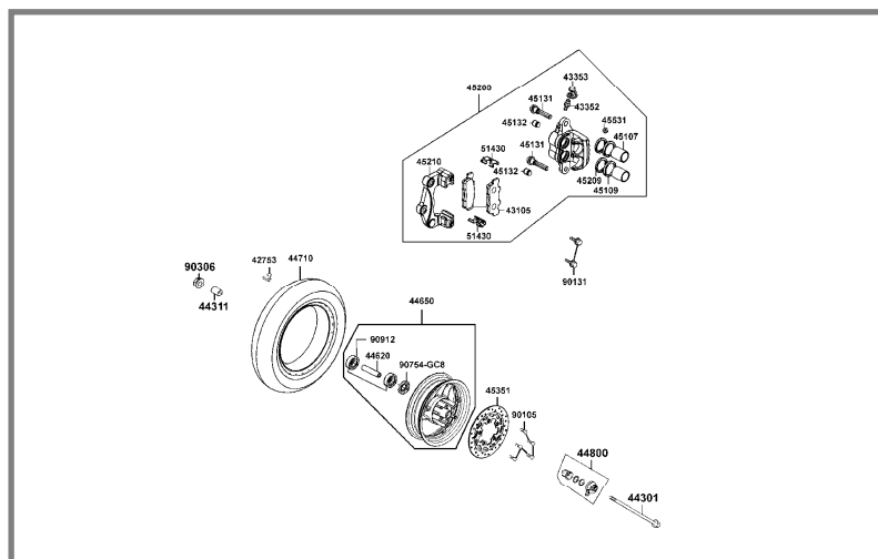
F07 RUEDA DELANTERA (Pág. 81)
