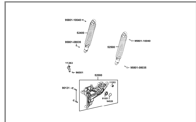
F16 AMORTIGUADORES TASEROS (Pág. 111)
