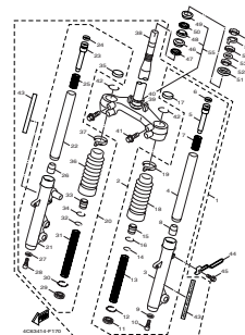
Fig. 17 前叉 ..... 59
