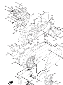
Fig. 9 曲軸箱 ..... 29
