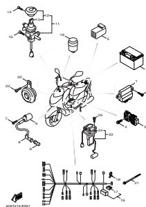
Fig. 35 電裝1 ..... 113
