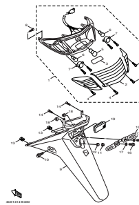
Fig. 33 後燈 ..... 109
