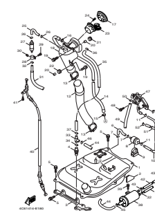
Fig. 18 汽油箱 ..... 65
