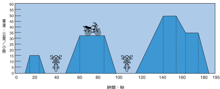
圖四、歐洲ECE-40行車型態
