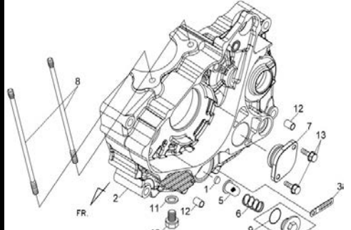
E18 L.CRANK CASE COMP
