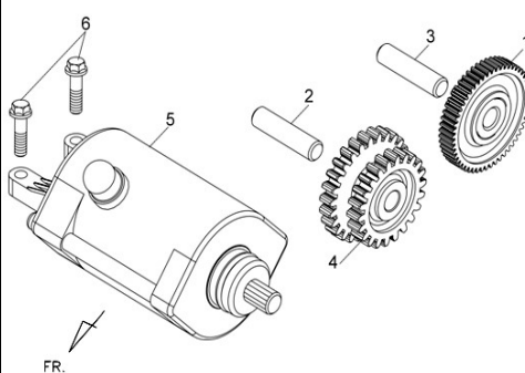
E20 START.MOTOR&START GEAR
