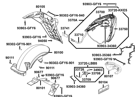
F18 後燈 ● 後土除
