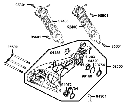
F16 後避震器
