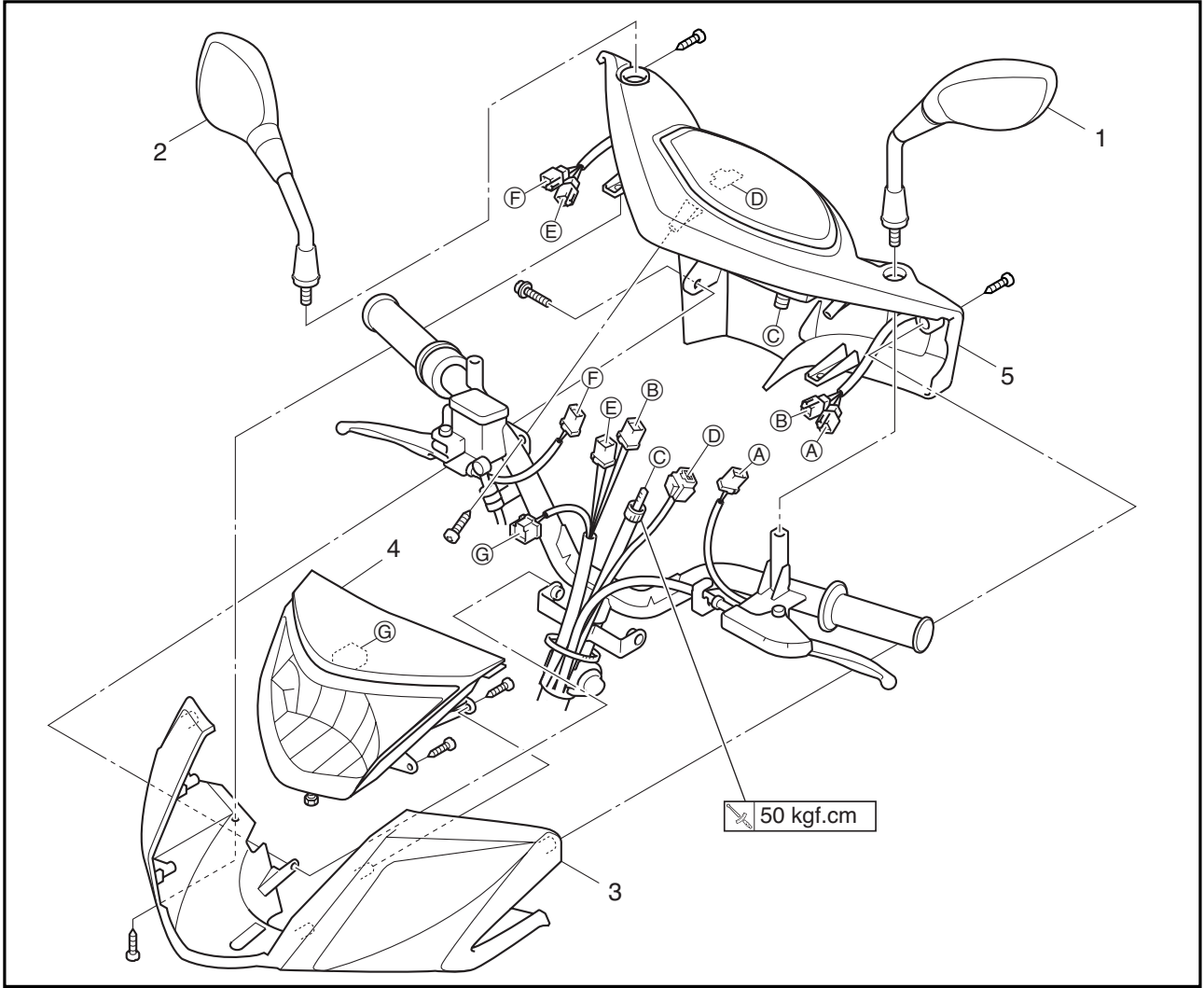
把手蓋1、2 (17C1)
