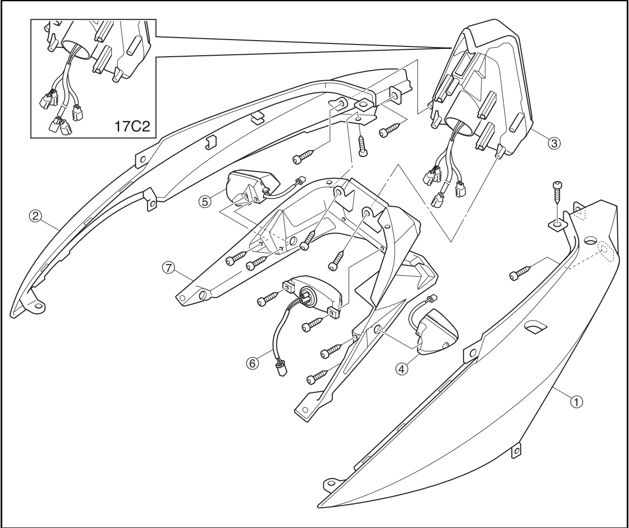
側蓋總成
