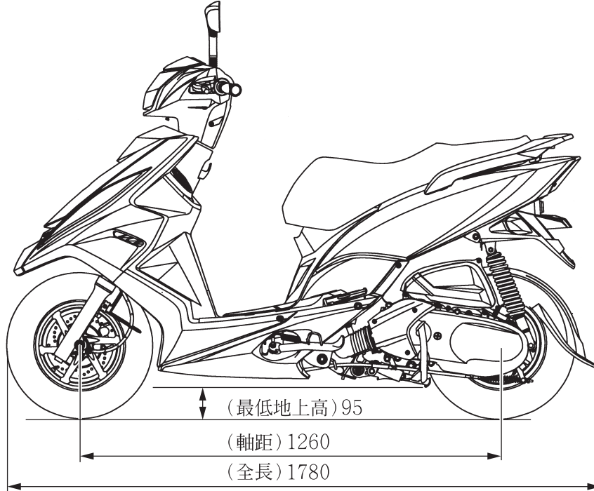
側面圖
